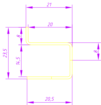
Проекция нижних лапок
